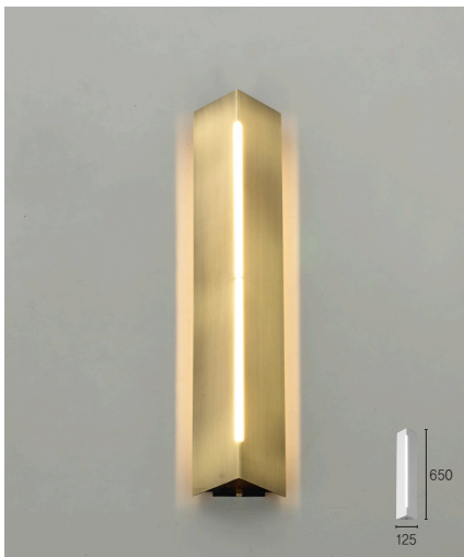
낭트 B/R (소) 신브 SIZE W125×D65×H670 뒷 판 W70×D25×H650 LAMP LED11W
