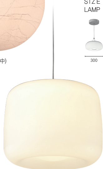
네스트 1등 P/D (3호) SIZE W260×H200 LAMP LED 24W (4000K)
