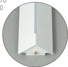
낭트 B/R (소) 신브 SIZE W125×D65×H670 뒷 판 W70×D25×H650 LAMP LED11W
