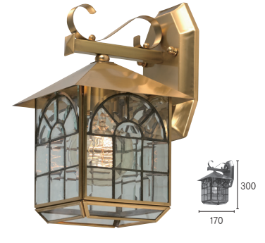
베로나 B/R (5호) B타입 (황동신주)(외부가능) SIZE W170×D190×H300 LAMP E26×1
