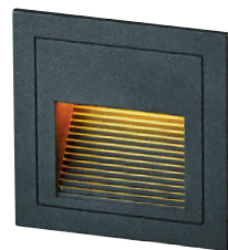
외부 키티 발목등 사각 1호 (매입) (흑색, 다크그레이, 백색) SIZE W85×H85 LAMP LED 3W (전구색) IP 65
