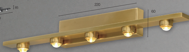
갤러리 웨이브 5등 B/R (황동신주) SIZE W500×D60×H85 LAMP LED 10W (3000K)
