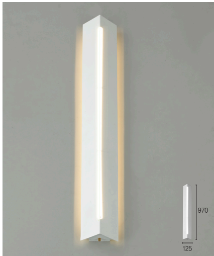
낭트 B/R (대) (화이트) SIZE W125×D65×H970 뒷 판 W70×D25×H950 LAMP LED15W
