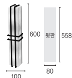
클라우드 B/R (A) (외부가능) SIZE W100×D100×H600 LAMP E26×4
