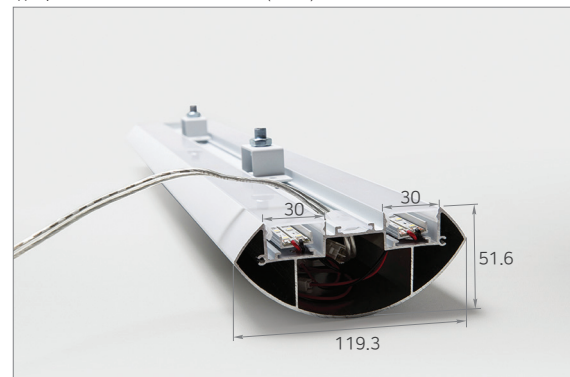
라인120x52 안정기 내장형 | 업라이트 규격 : W 119.3 x H 51.6 x L(mm)
