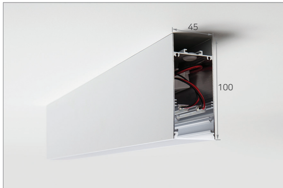
라인45x100 안정기 내장형 규격 : W 45 x H 100 x L(mm)
