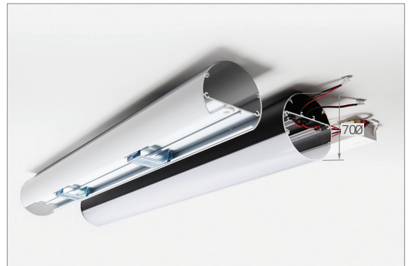
라인70 \varnothing 파이프형 안정기 외장형 규격 : 70 \varnothing x L(mm)
