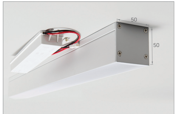
라인50x50 안정기 외장형 규격 : W 50 x H 50 x L(mm)
